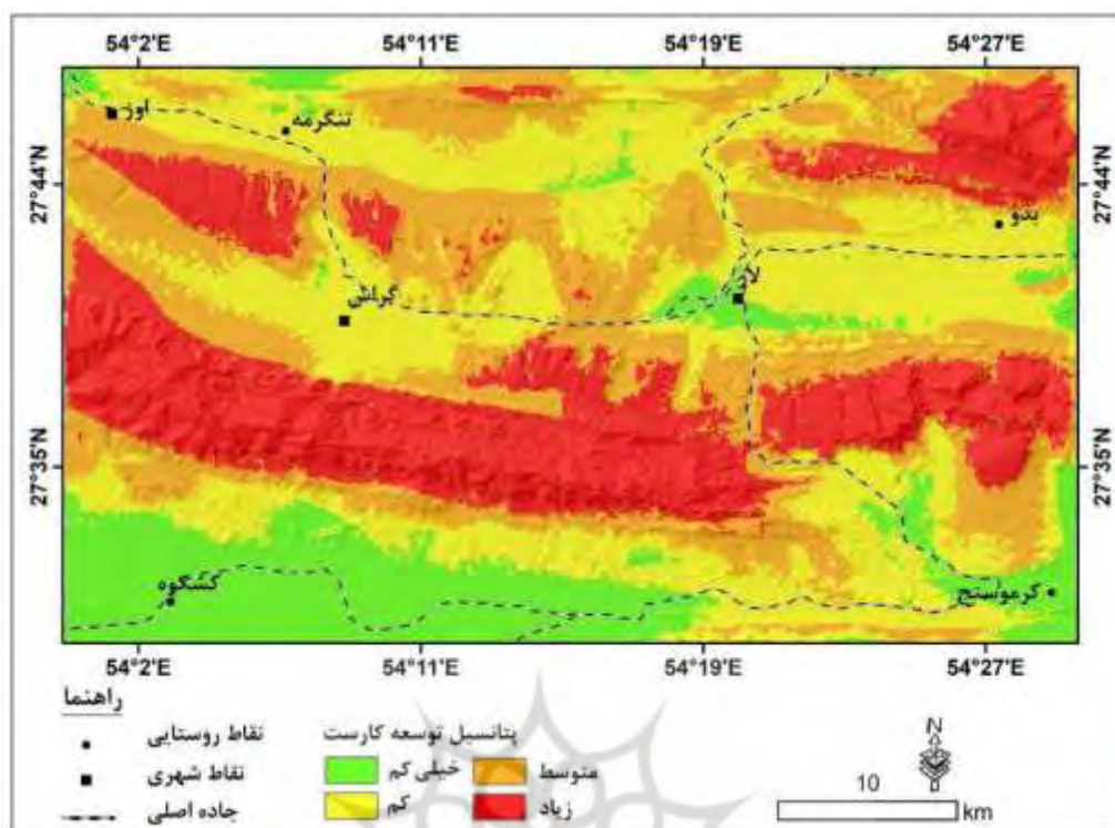
شکل (۴): نقشه پتانسیل توسعه فرایندهای کارستیک (محدوده اوز تا کرموستاج استان فارس)
