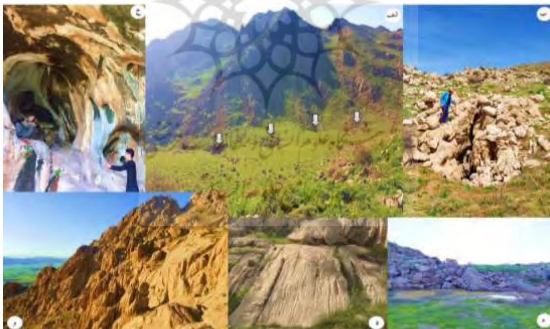
شکل ۹- الف: فروچاله‌های کارستی توده کارستی شاهو و پونورهای کف آن، ب: نمونه‌ای از دولین‌ها در ارتفاع ۳۱۴۰ متری شاهو، ج: فراوانی غار در دامنه‌های شاهو د: کف دولین کارستی در ارتفاع ۳۲۱۰ متری، ه: کارن‌های شیباری که به عنوان هدایت‌کننده آب‌های سطحی عمل می‌کنند، و: درز و شکاف و کارن‌های شیباری فراوان در آهک بیستون (منبع: نگارندگان)
