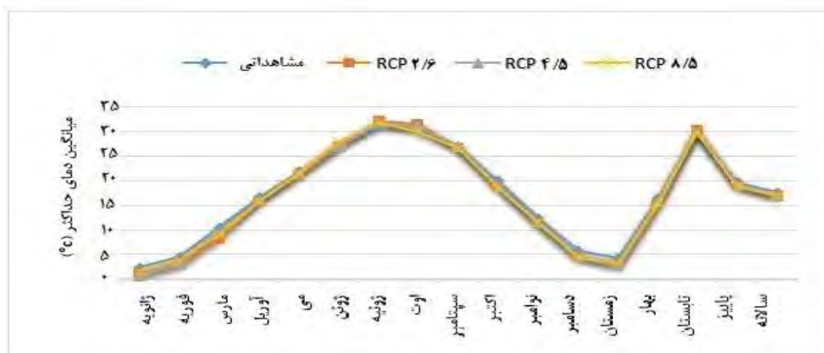
شکل ۴. نمودار مقایسه‌ای مقادیر مشاهداتی و شبیه‌سازی شده براساس سناریوهای مدل CanESM2 (۱۹۶۱-۲۰۰۵)
