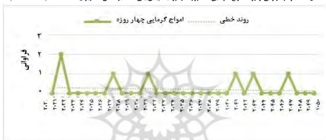
شکل ۹. نمودار فرآوانی و روند امواج گرمایی چهار روزه در ارومیه، پیش‌بینی شده براساس سناریوی RCP ۸/۵ (۲۰۲۰-۲۰۵۰)
