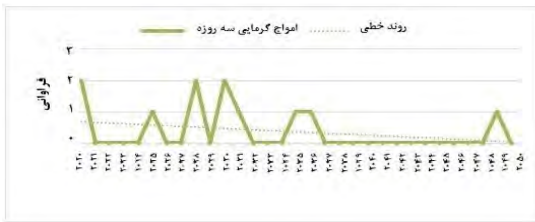
شکل ۸. نمودار فرآوانی و روند امواج گرمایی سه روزه در ارومیه، پیش‌بینی شده براساس سناریوی RCP ۸/۵ (۲۰۲۰-۲۰۵۰)
