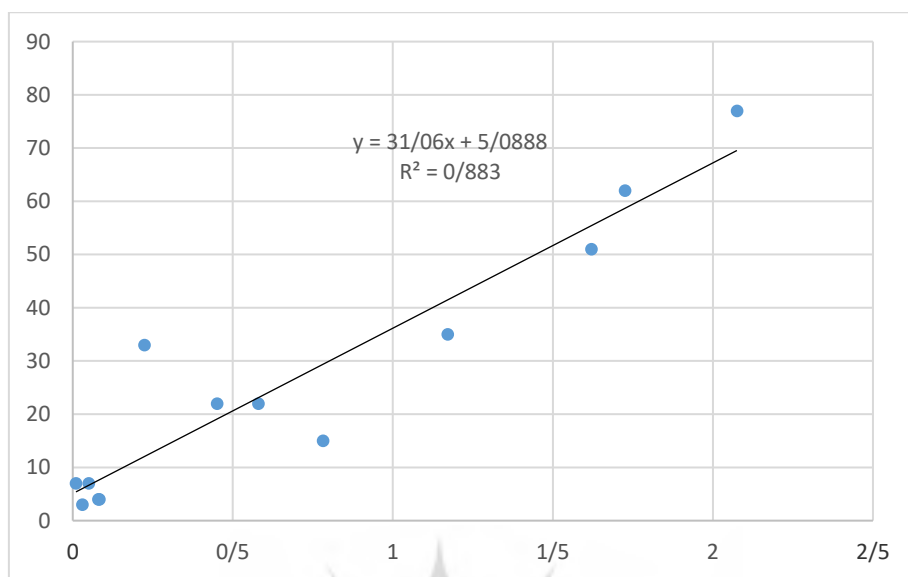
شکل ۹: نمودار ضریب همبستگی بین میزان فروروشست زمین و افت سطح آب چاه‌ها
