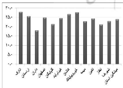
شکل (۱۳) میانگین بیشینه دمای
