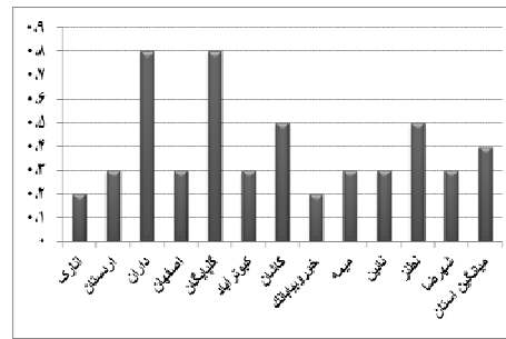
شکل (۱۴) میانگین بارش ایستگاه‌های همدید
