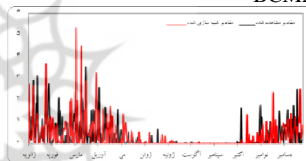
شکل (۶) مقایسه مقدار تابش دیده بانی شده و شبیه سازی شده با مدل B1-BCM2
