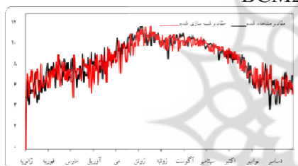
شکل (۵) مقایسه مقدار بارش دیده بانی شده و شبیه سازی شده با مدل B1-BCM2
