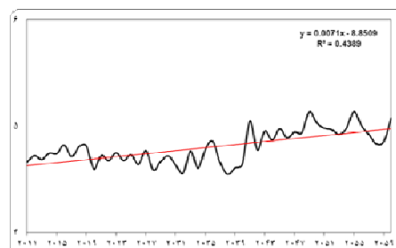
شکل (۸) مدل سازی دمای بیشینه اصفهان در دوره ۲۰۱۱-۲۰۶۰ با مدل B1-BCM2
