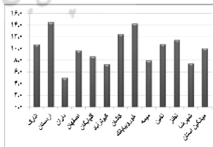
شکل (۱۲) میانگین کمینه دمای ایستگاه‌های
