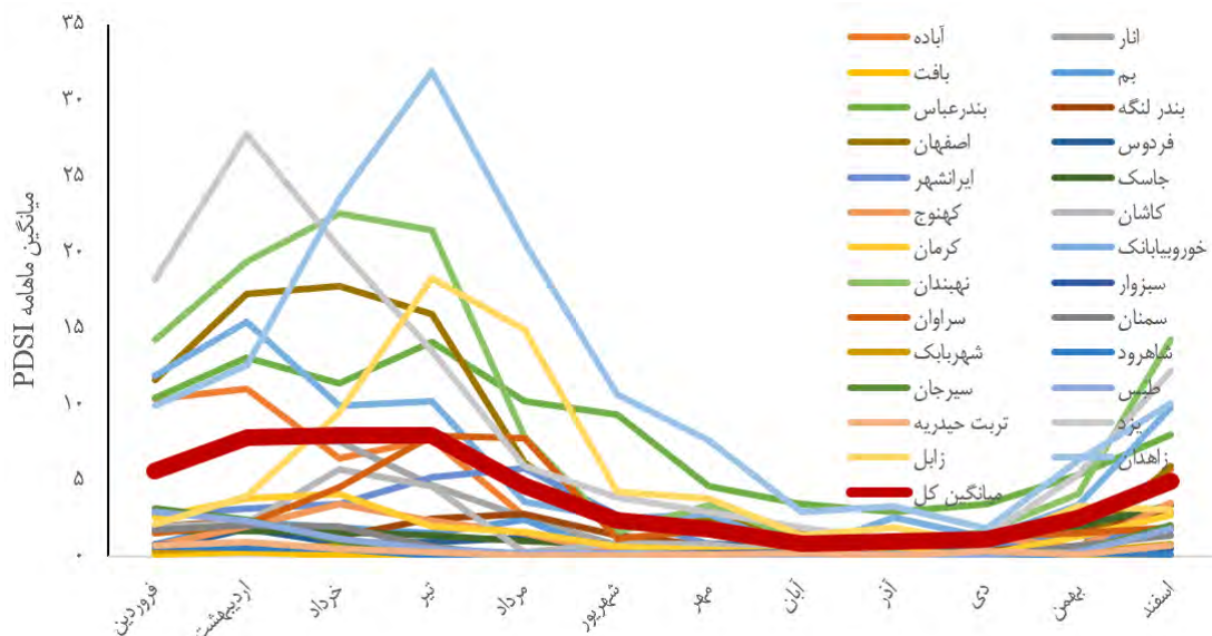
شکل ۴. مقادیر میانگین ماهانه PDSI طی سال‌های ۱۳۷۹ تا ۱۳۹۷ در ایستگاه‌های مطالعاتی
