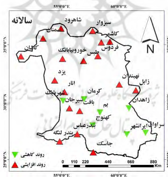
شکل ۳. روند تغییرات سالانه شاخص غبارآلودگی توفان در ایستگاه‌های مطالعاتی واقع در مناطق خشک ایران طی دوره آماری ۱۳۷۹ تا ۱۳۹۷
