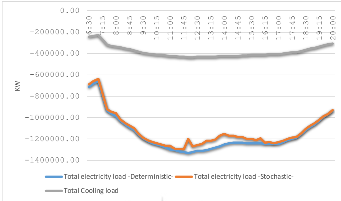
شکل ۱۲: مصرف برق در حالت پایه و مقایسه بار الکتریکی تصادفی و قطعی (پیک روز)
