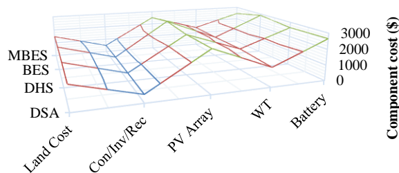
شکل (۱۱): هزینه قطعات (LPSP = ۰٪)
