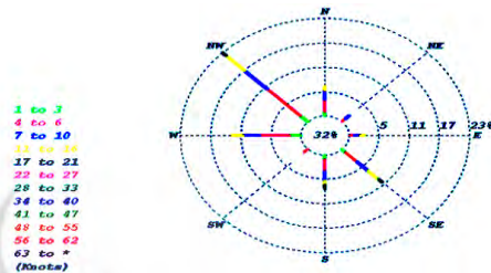
شکل ۳) گلباد سالانه ایستگاه هواشناسی آبادان
