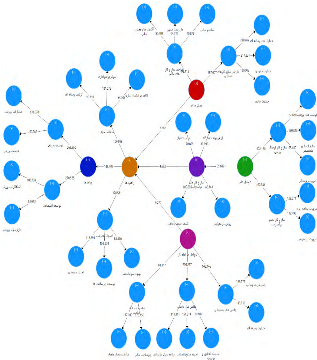
شکل ۲- مدل نهایی پژوهش در حالت مقادیر معناداری (T. Value) Figure 2- The final research model in the mode of significant values (T. Value)
