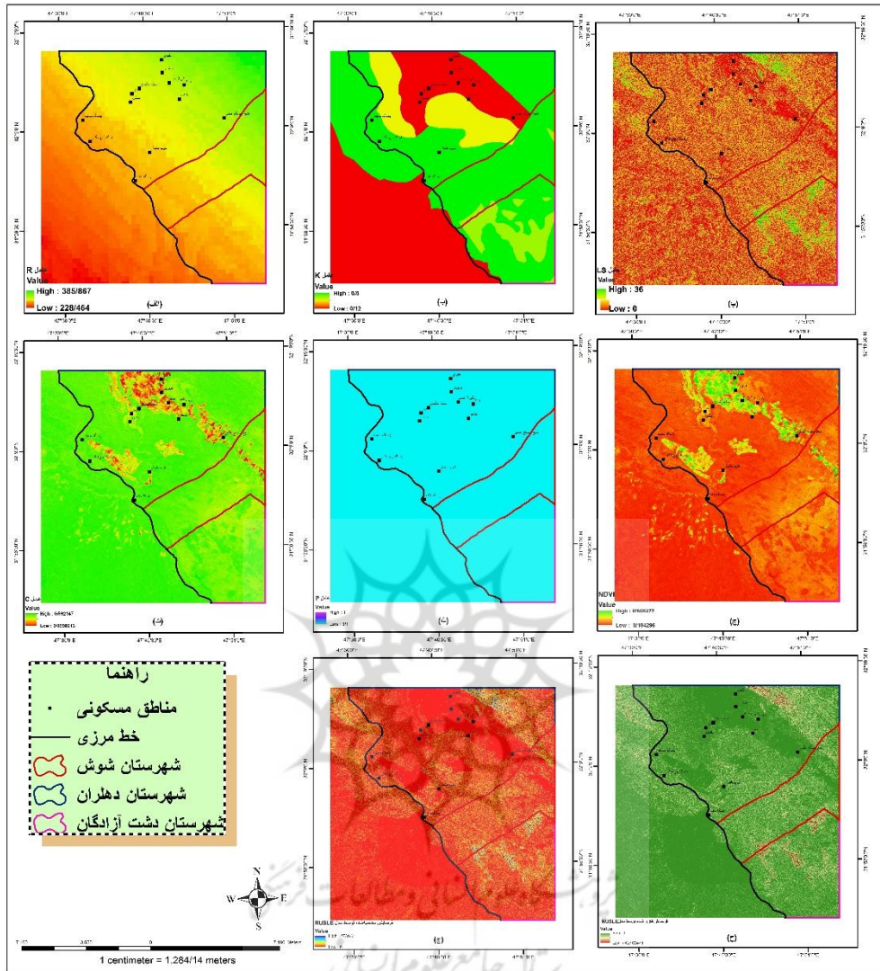
شکل (۶) نقشه فرسایش و عوامل دخیل در فرسایش خاک (الف: عامل R، ب: عامل K، پ: عامل عامل LS، ت: عامل C، ث: عامل P، ج: عامل NDVI، چ: فرسایش محاسبه شده توسط مدل RUSLE، ح: فرسایش فازی شده توسط مدل RUSLE)
