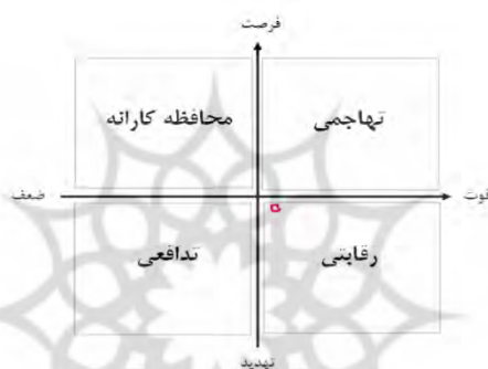
شکل ۱: حوزه‌های ماتریس SWOT
