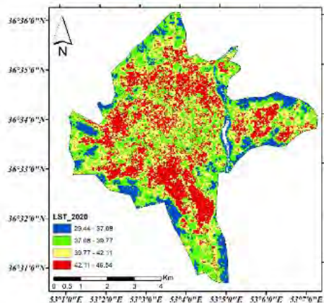
شکل ۳- نقشه دمای سطح زمین، شهر ساری - در تاریخ ۱۳/۰۶/۱۹۹۰، ۱/۰۶/۲۰۰۰، ۴/۰۶/۲۰۱۰، ۶/۰۶/۲۰۲۰
