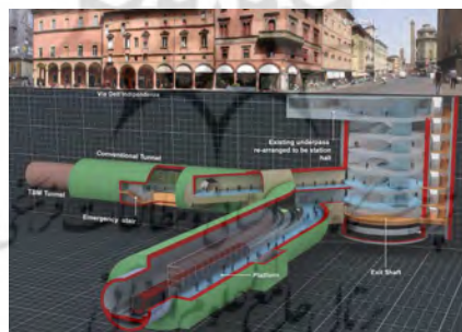
شکل ۸- دید سه بعدی به فضاهای زیرسطحی ایستگاه مترو میدان بولونا در شهر سان مارینو ایتالیا
