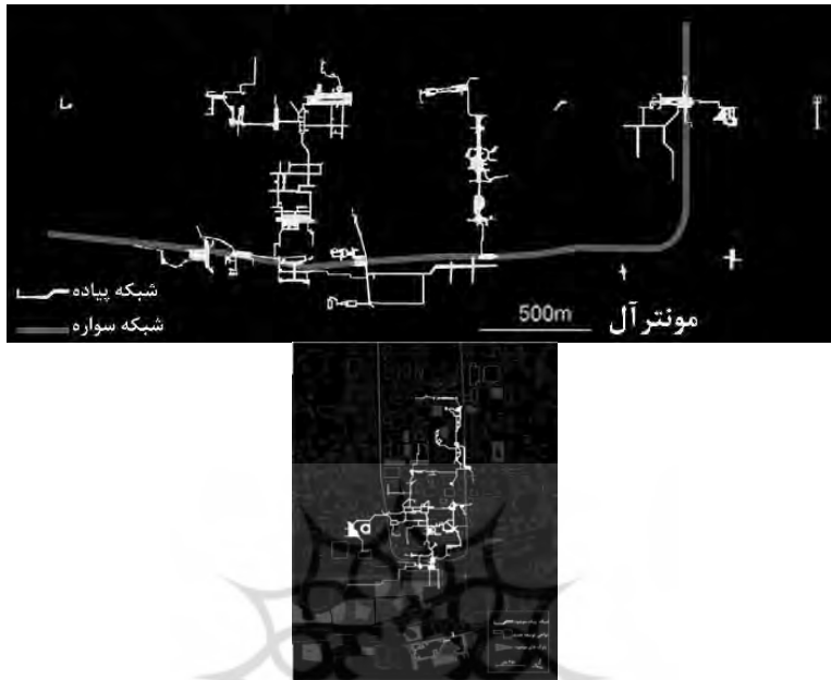
شکل ۱۲- پلان شبکه زیرزمینی شهر مونترال و تورنتوی کانادا (Be langer, 2007)
