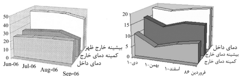
شکل ۱۰- مقایسه دمای هوای داخل و خارج شوادان در تابستان و زمستان
