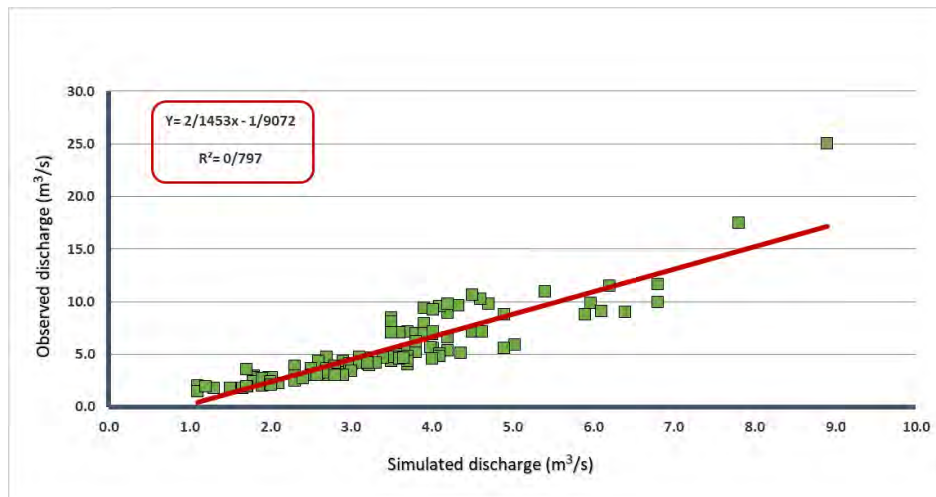
شکل ۵. نمودار رگرسیون خطی میان دبی مشاهده‌ای و شبیه‌سازی‌شده - واسنجی مدل AWBM
