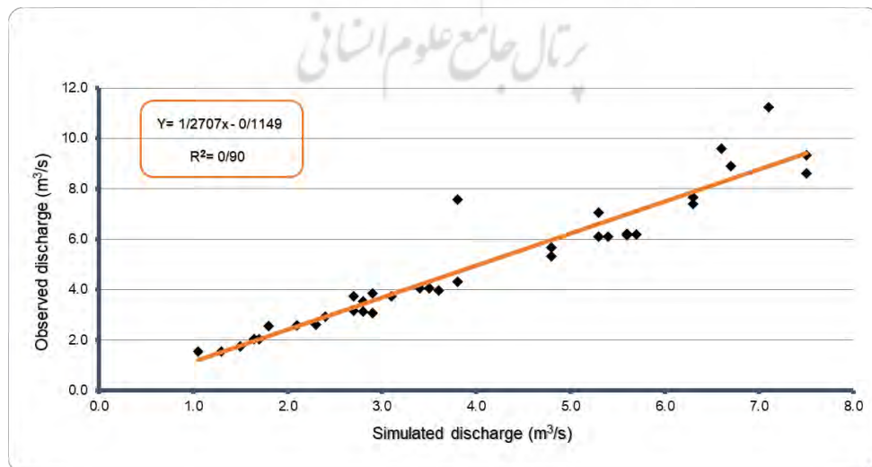
شکل ۷. نمودار رگرسیون خطی بین دبی مشاهده‌ای و شبیه‌سازی‌شده - اعتبارسنجی مدل AWBM
