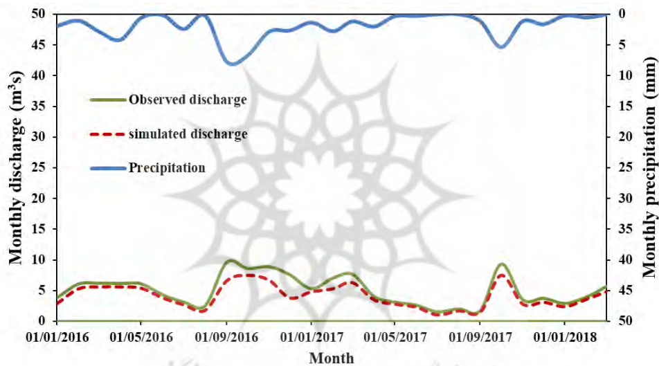
شکل ۶. مقادیر ماهانه دبی مشاهده‌ای و شبیه‌سازی‌شده در مرحله اعتبارسنجی مدل AWBM
