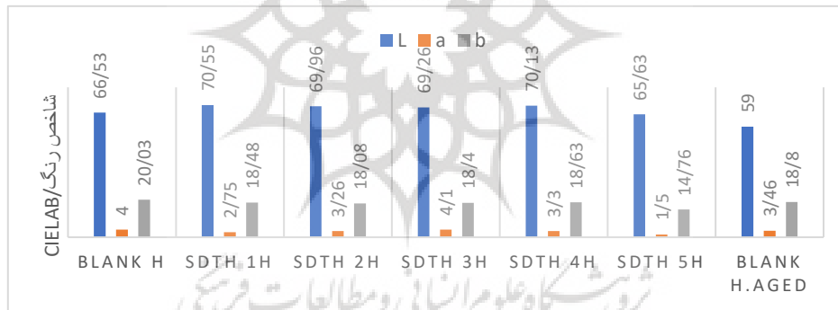
شکل ۱۰: مؤلفه‌های رنگی نمونه‌های تاریخی درمان شده با دی‌تیونیت سدیم پس از کهنه‌سازی. Fig. 10: Color parameters of historical samples treated with sodium dithionite after aging.
