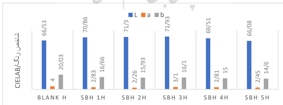
شکل ۱۱: مؤلفه‌های رنگی نمونه‌های تاریخی درمان شده با بوروهیدرید سدیم قبل از کهنه‌سازی. Fig. 11: Color parameters of historical samples treated with sodium borohydride before aging.
