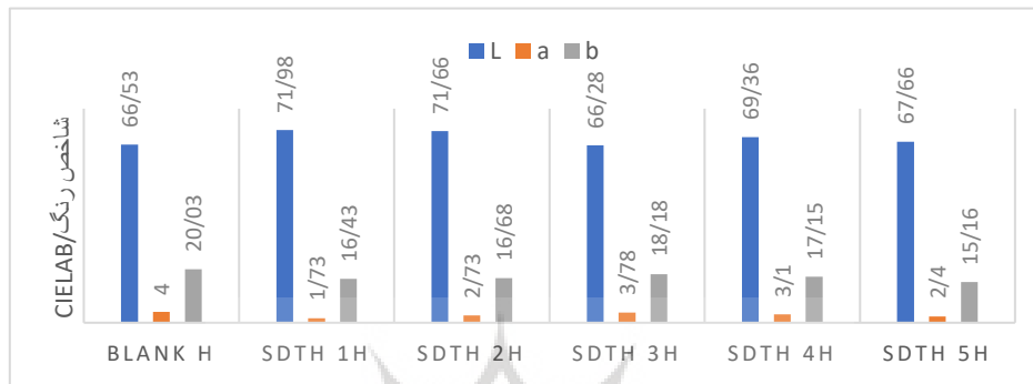
شکل ۹: مؤلفه‌های رنگی نمونه‌های تاریخی درمان شده با دی‌تیونیت سدیم قبل از کهنه‌سازی. Fig. 9: Color parameters of historical samples treated with sodium dithionite before aging.
