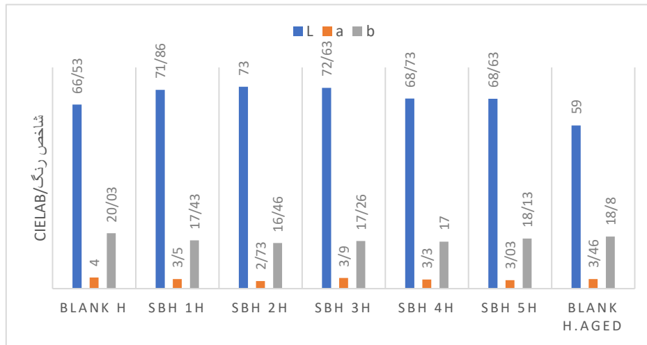
شکل ۱۲: مؤلفه‌های رنگی نمونه‌های تاریخی درمان شده با بوروهیدرید سدیم پس از کهنه‌سازی. Fig. 12: Color parameters of historical samples treated with sodium borohydride after aging.
