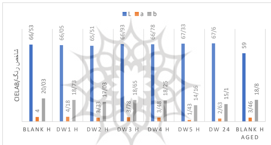
شکل ۱۳: مؤلفه‌های رنگی نمونه‌های تاریخی درمان شده با آب مقطر قبل از کهنه‌سازی. Fig. 13: Color parameters of historical samples treated with distilled water before aging.
