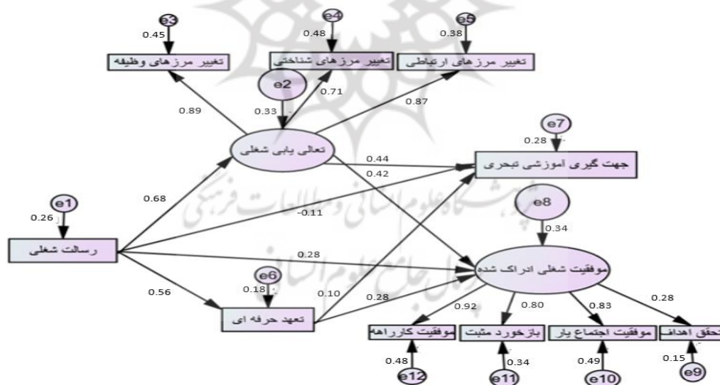
شکل ۱. ضرایب استاندارد مسیرهای مستقیم
