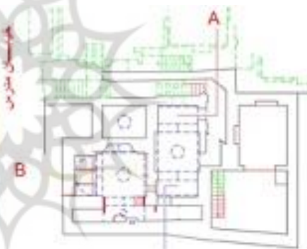
شکل (۹). پلان و بینه حمام بیگلری (نگارندگان، ۱۳۹۹)
