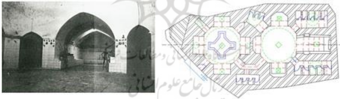
شکل (۱۱). پلان و گرمخانه حمام معاون (منبع: آرشیو میراث فرهنگی استان کرمانشاه، ۱۳۹۹)
