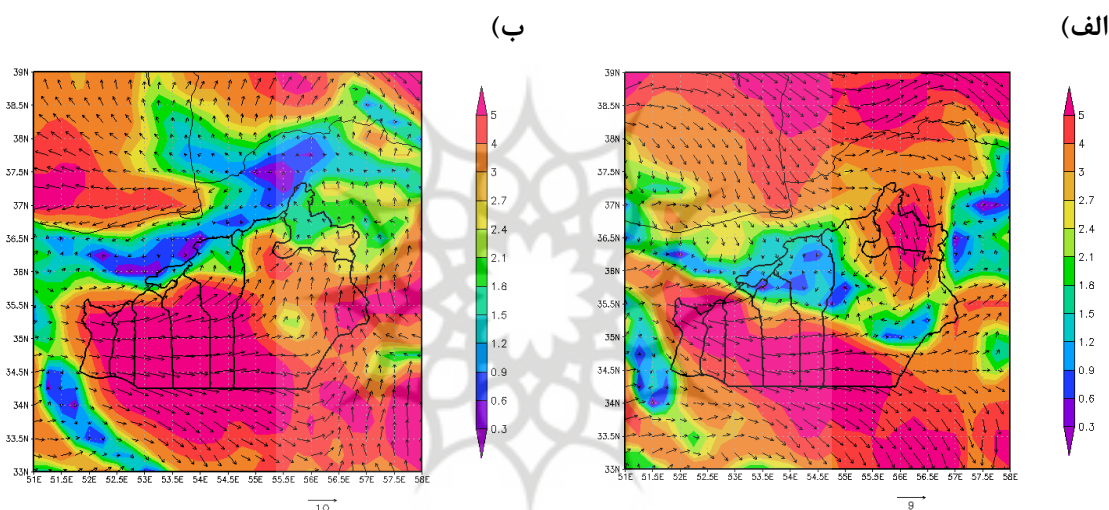
شکل (۱۰). سرعت و جهت باد ۱۰ متری استان سمنان و استان‌های مجاور در الف - ۱۴ مارس ۲۰۰۸ ساعت ۱۲UTC ب- ۲۱ آوریل ۲۰۱۵ ساعت ۱۲UTC
