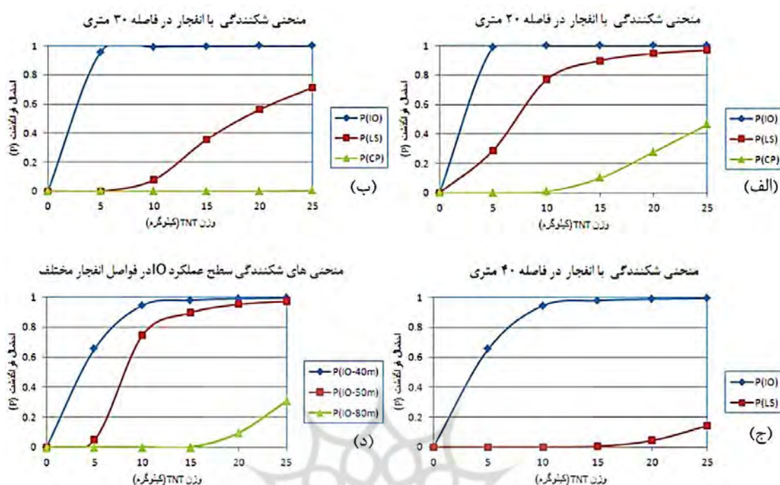
شکل ۷: منحنی‌های شکنندگی انفجار در فاصله‌های (الف) ۲۰ متری، (ب) ۳۰ متری، (ج) ۴۰ متری، (د) سطح عملکرد IO در فواصل مختلف (نگارندگان)
