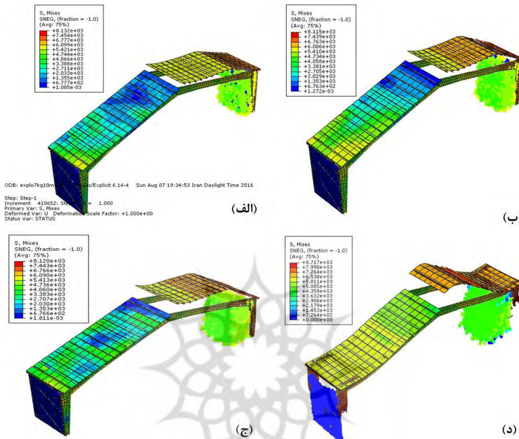
شکل ۳: تغییر شکل سازه پس از انفجار. الف) ۷٫۵ کیلوگرم معادل TNT ماده منفجره، ب) ۲۵ کیلوگرم معادل TNT ماده منفجره، ج) ۳۵ کیلوگرم معادل TNT ماده منفجره، د) ۵۰ کیلوگرم معادل TNT ماده منفجره؛ در فاصله ۱۰ متری بیرون سازه (نگارندگان)
