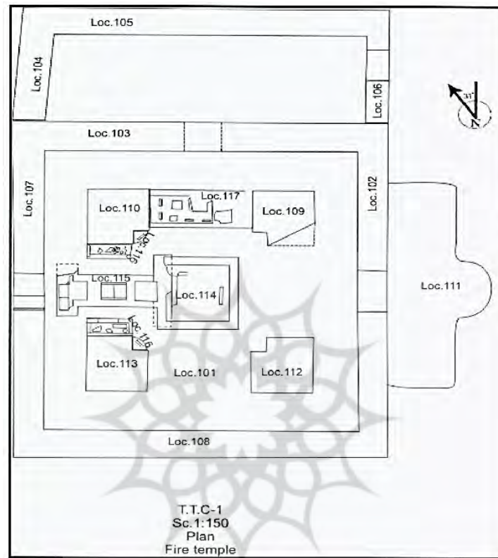
شکل ۶: پلان آتشکده شیان (سازمان میراث فرهنگی کرمانشاه، پرونده ثبتی آتشکده شیان). جدول ۱: راهنمای پلان آتشکده شیان (نگارنده).
