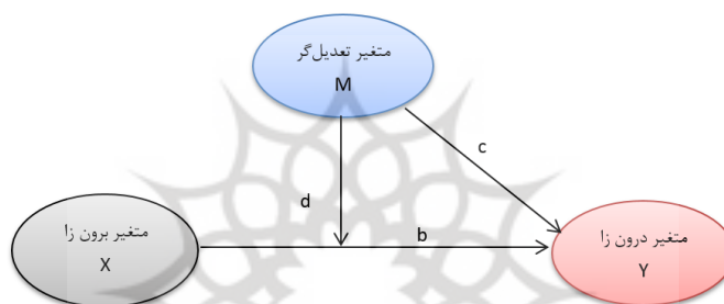
شکل ۱. مدل ساختاری با یک متغیر تعدیل کننده
