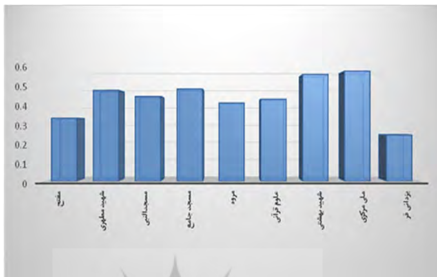
نمودار ۱- نزدیکی تا گزینه ایدئال
