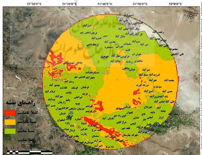
شکل ۲۱- پهنه‌های مناسب جهت اسکان موقت
