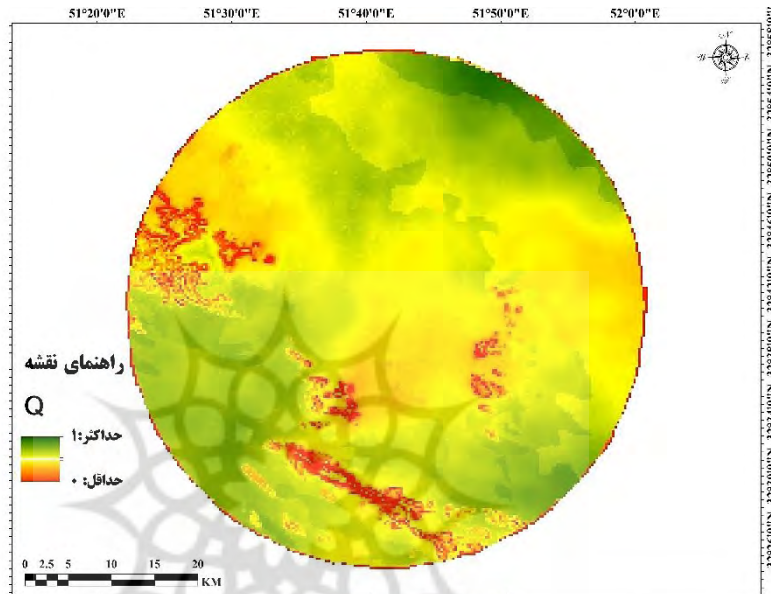
شکل ۲۰- شناسایی مناسب‌ترین پهنه‌ها و اراضی جهت اسکان موقت با مدل ویکور
