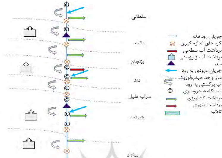
شکل ۲- الگوی شماتیک حوضه آبریز جازموریان غربی
