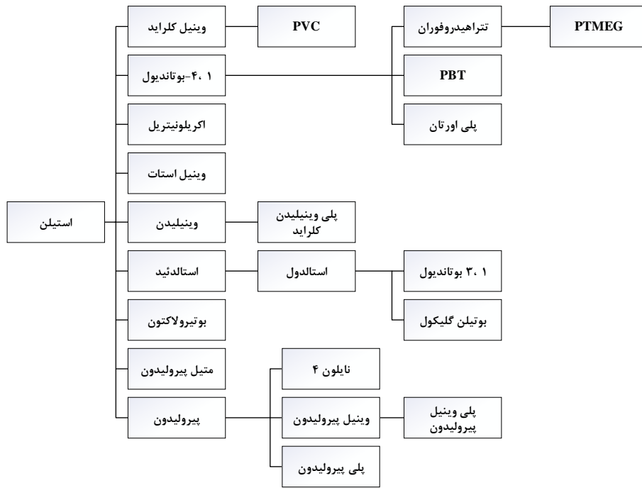
شکل ۵: زنجیره ارزش استیلین [۵۴]
