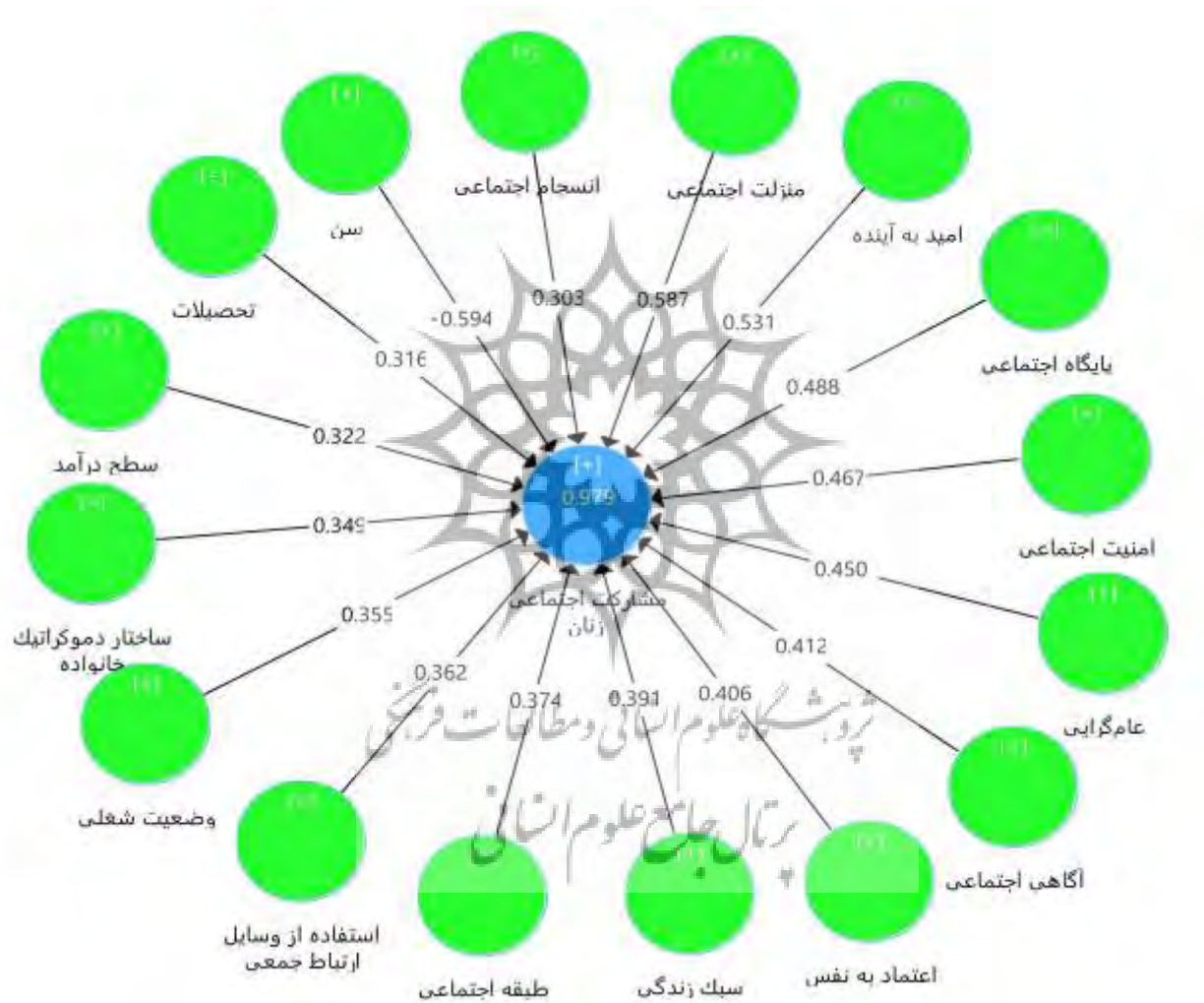
شکل ۱- ضرایب مسیر
