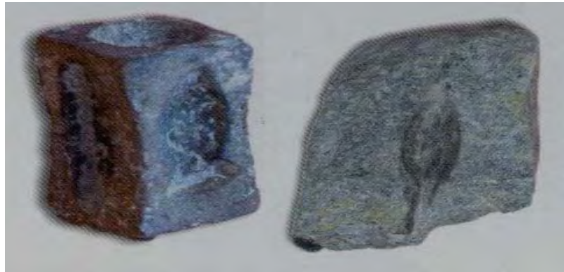
تصویر ۴: قالبهای سنگی سرپیکان، مکشوفه از محوطه های باستانی شرق آناتولی، محل نگهداری: موزه باستان شناسی سینوپ و سامسون ترکیه (برگرفته از ۲۸: ۲۰۰۴، Bilgi).
