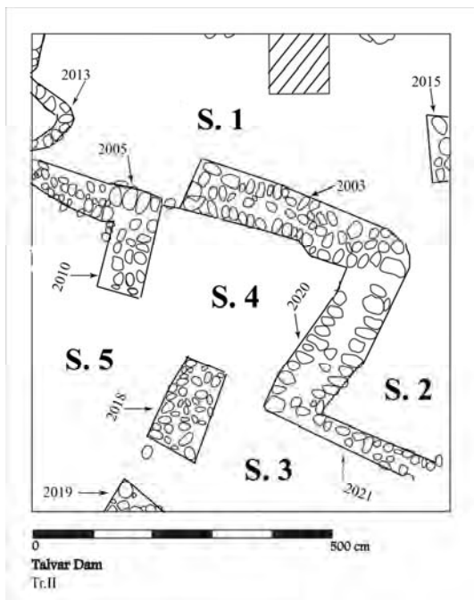
پلان ۱: پلان نهایی ترانسه II.
