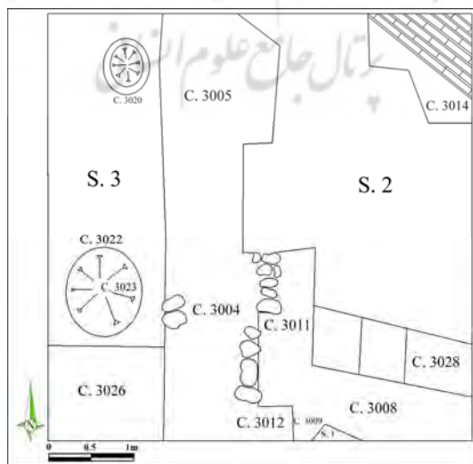
پلان ۲: پلان نهایی ترانسه III.
