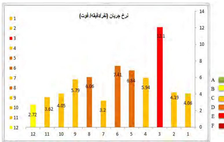
شکل ۷. سطح سرویس معابر بر اساس نرخ جریان (نفر/دقیقه/فوت)
