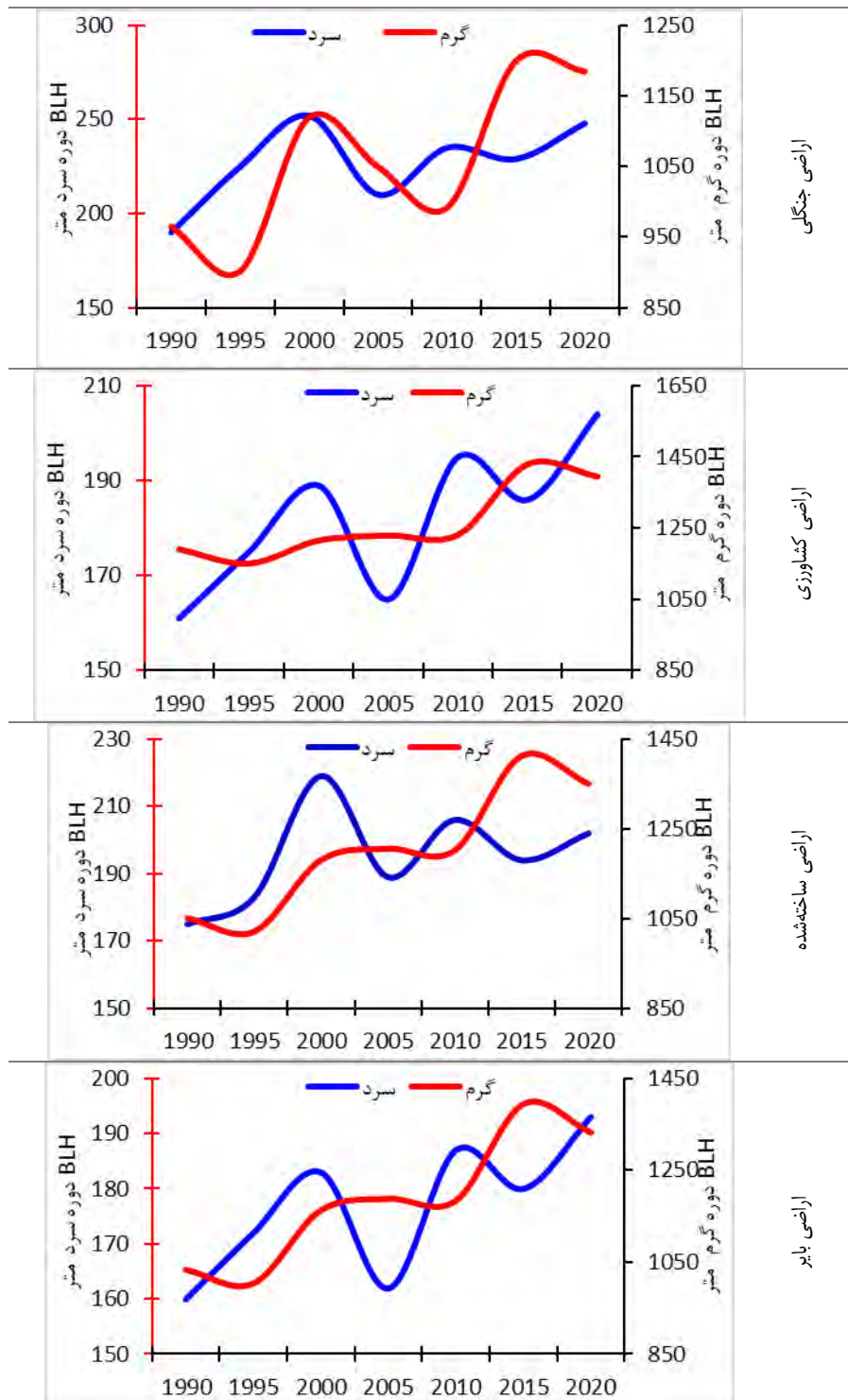
شکل ۶. روند دوره‌ای تغییرات میانگین فضایی شاخص ارتفاع لایه مرزی BLH (مستخرج از پایگاه ERA5 با رزولوشن فضایی ۰/۲۵ درجه قوسی) در سطح هر کدام از طبقات پوشش اراضی استان لرستان طی دوره گرم و سرد سال دوره آماری ۱۹۹۰-۲۰۲۰
