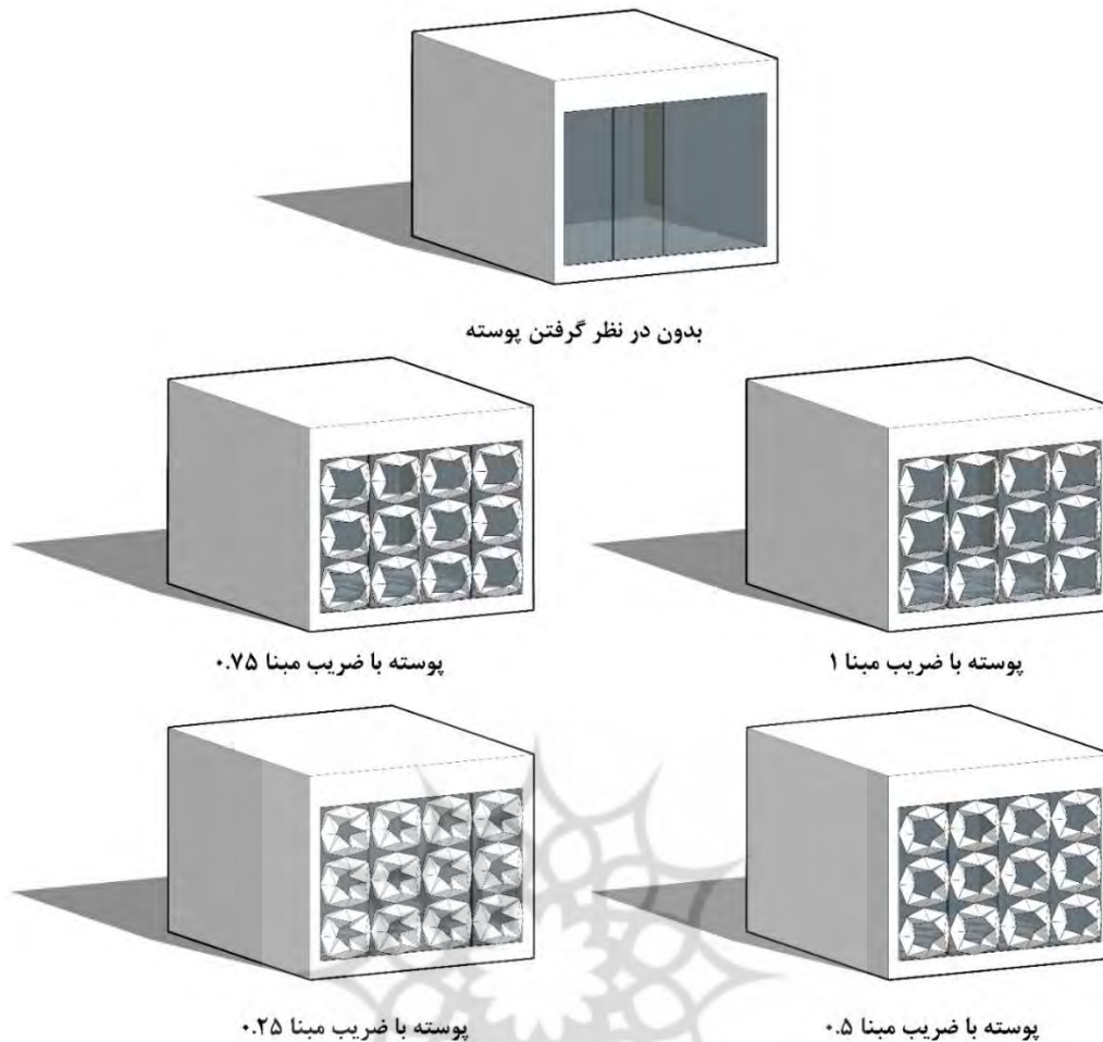
تصویر ۹. پنج حالت مختلف از بازشدگی پوسته دوم به جهت آنالیز نور روز (مأخذ: نگارندگان)
