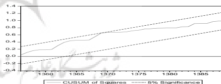
شکل ۴: نمودار آزمون CUSUM و CUSUMSQ در مدل سوم
