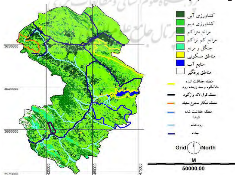
شکل ۳: نقشه کاربری و پوشش اراضی زیرحوضه آب‌خیز پلاسجان در سال ۱۳۹۶ (راهداری و همکاران، ۱۳۹۶ و نتایج تحقیق حاضر)
