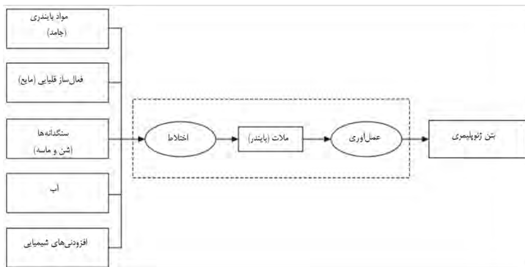
شکل ۷. مرز سیستم برای شناخت فرآیندهای مربوط به تولید
