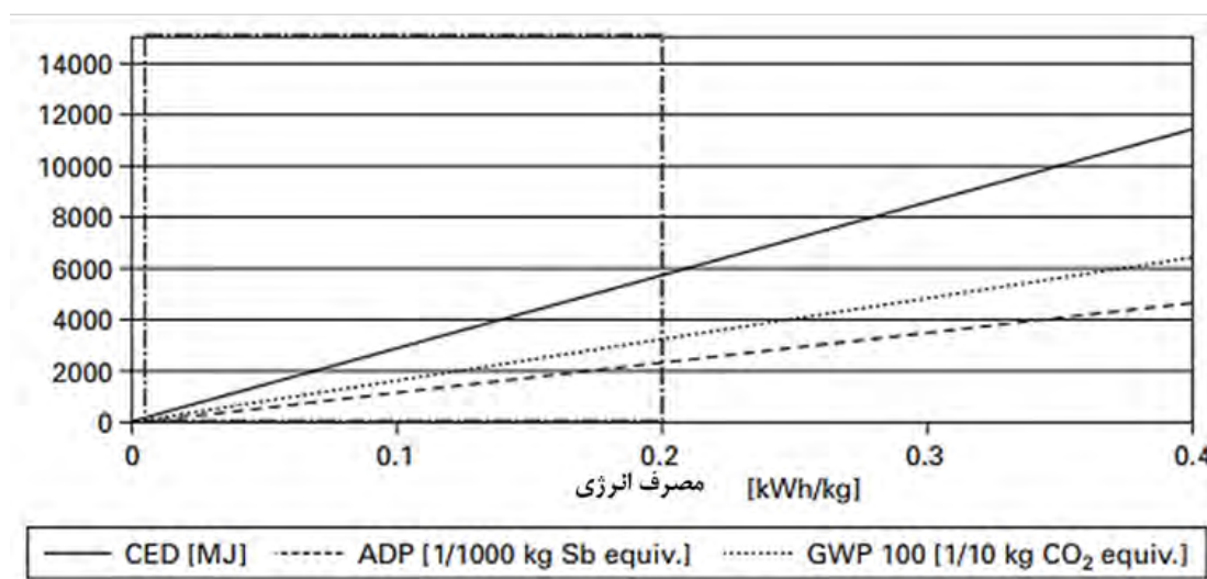
شکل ۸. تاثیر عمل‌آوری حرارتی (مصرف انرژی الکتریکی) بر اثرات شاخص‌های محیط زیستی (تقاضای تصاعدی انرژی)، GWP (پتانسیل گرمایش جهانی)، ADP (پتانسیل تخریب منابع غیرزیستی)
