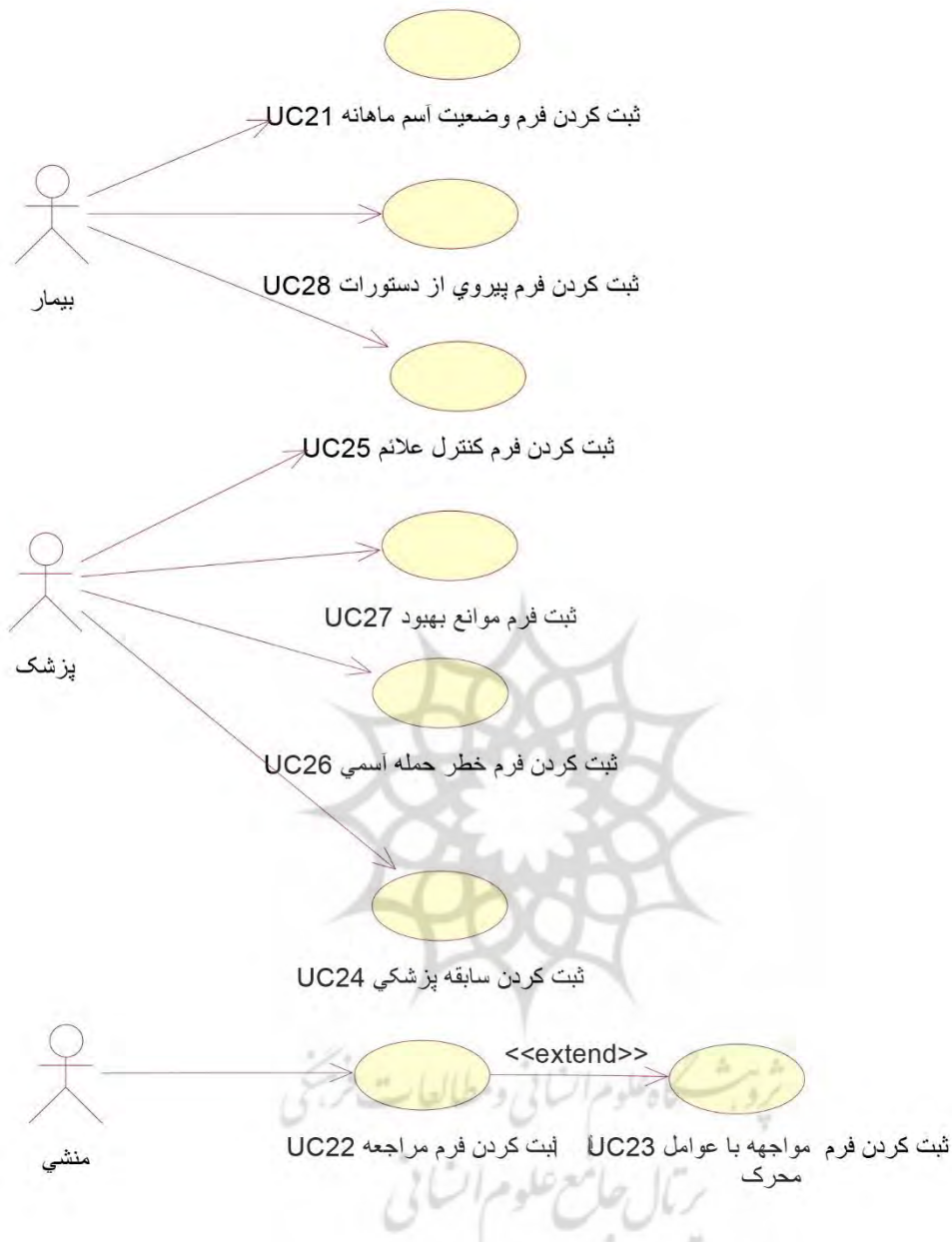
شکل 5: نمودار مورد - کاربرد کسب و کار ثبت داده در سامانه
