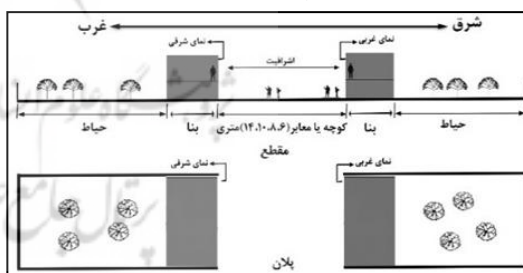
ت ۹. نحوه استقرار واحدها در ارتباط با معابر و حیاط در بافت قدیمی روستای سپورغان (مأخذ: نگارندگان).
