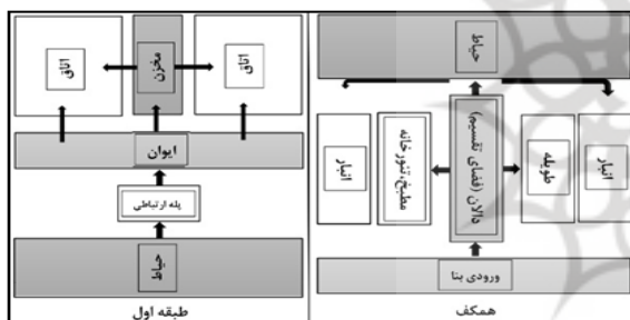
ت ۱۱. دیاگرام عمومی بناهای سنتی روستای سپورغان (مأخذ: نگارندگان).
