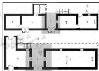
ت ۱۹. نمونه‌ای از پلان ساختار فضایی و کالبدی ورودی خانه‌های تاریخی و سنتی روستای سپورغان (مأخذ: نگارندگان).
