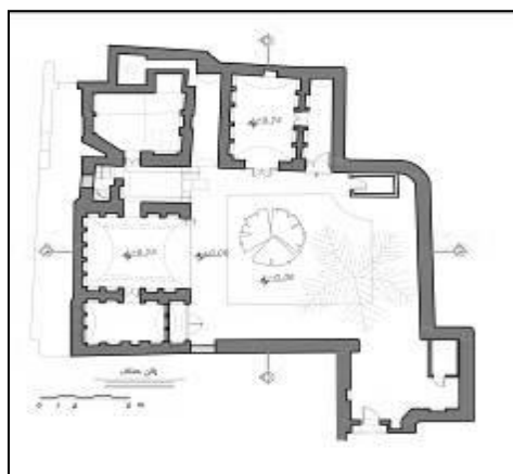
ت ۹. پلان یکی از خانه‌های قاجاری روستا (آرشیو اداره کل میراث فرهنگی، صنایع دستی و گردشگری استان یزد، ۱۳۹۱).
