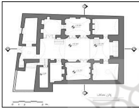
ت ۱۱. پلان یکی از خانه‌های دوره پهلویی (آرشو اداره کل میراث فرهنگی، صنایع دستی و گردشگری استان یزد، ۱۳۹۱)
