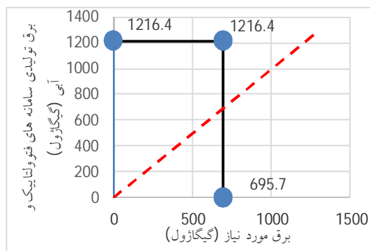
ن 6. مقایسه میزان برق مورد نیاز روستای نجوهران.
