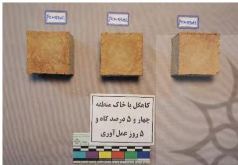
ت ۱۲. نمونه‌های کاهگل مکعبی برای تعیین مقاومت فشاری. مأخذ: نگارنده.
