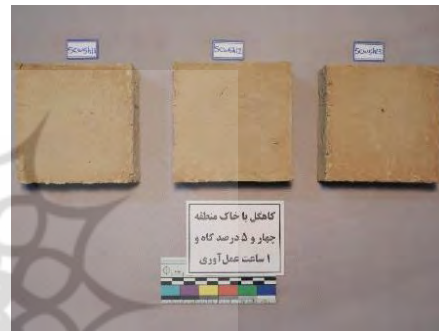
ت ۹. نمونه‌های کاهگل مکعب مستطیل. مأخذ: نگارنده.
