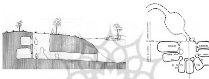
تصویر ۸. پلان و برش یک واحد مسکونی در ماتماتا، تونس (Source: Libaud, 1986, 121)
