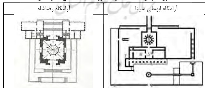
جدول ۳- پلان بناهای یادبودی دوره‌ی جدید، منبع: نگارندگان
