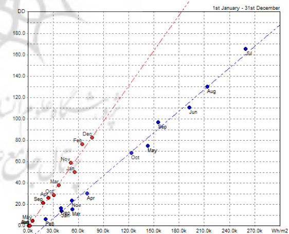
نمودار ۷- آنالیز حرارتی ساختمان (نرم افزار Ecotect) (نگارندگان)
