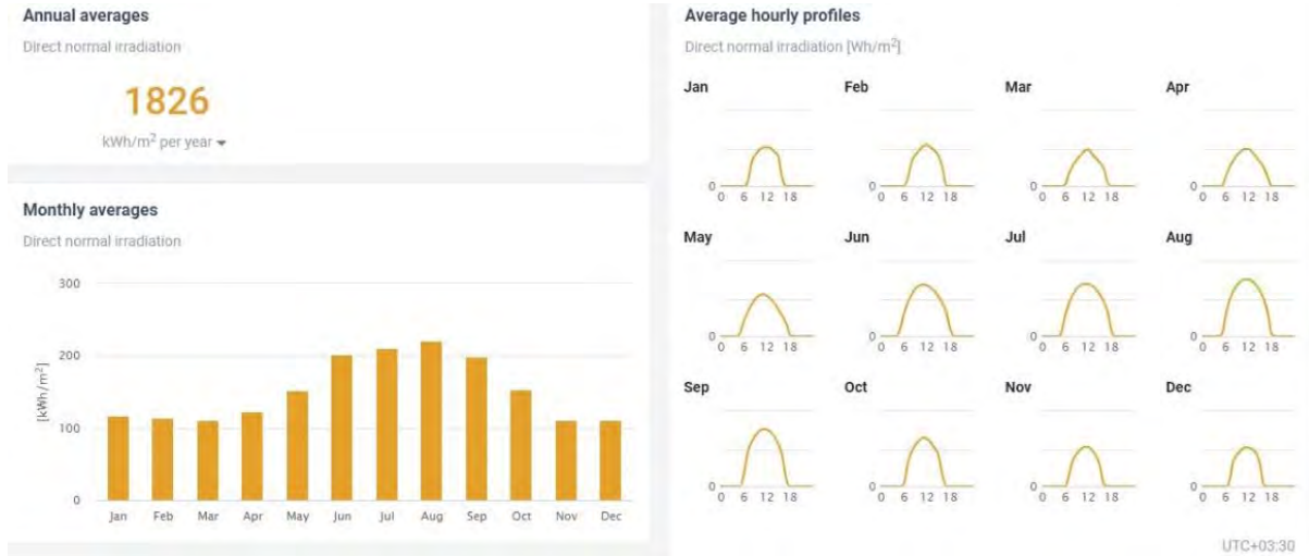
تصویر ۴- نمودار متوسط ساعتی، ماهانه و سالانه میزان دریافت تابش مستقیم خورشید در شهر مشهد (globalsolaratlas.info)
