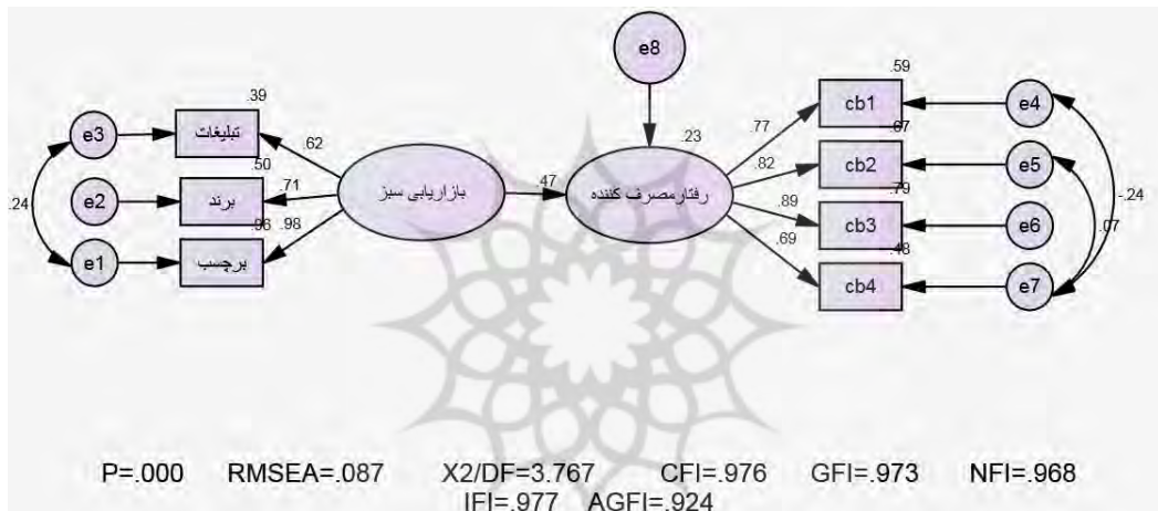
شکل ۱- الگوی کلی معادلات ساختاری پژوهش
