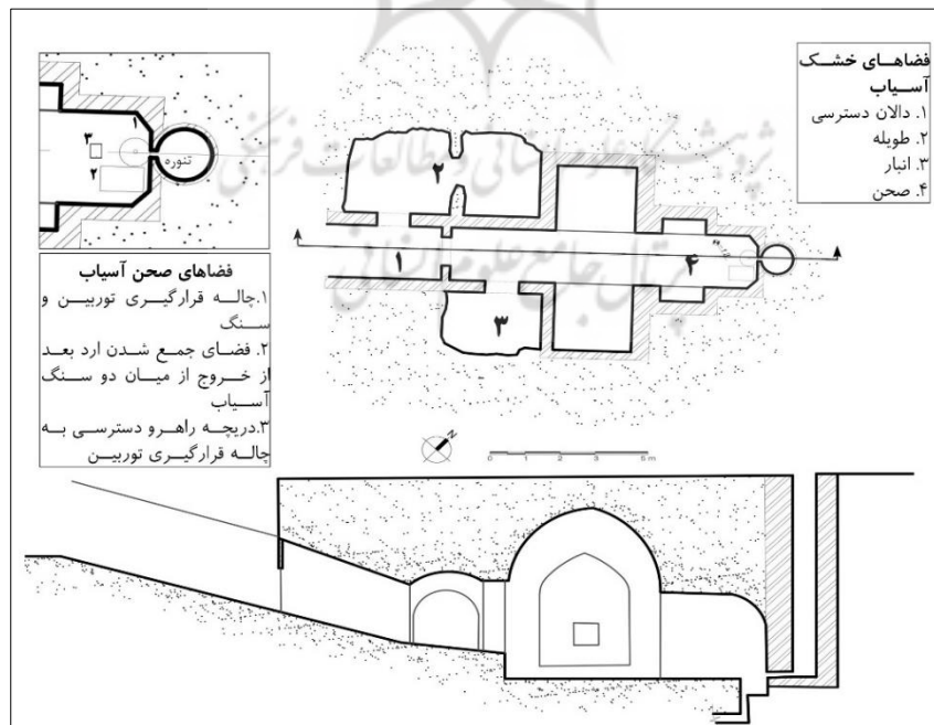
تصویر ۱۲. فضاهای کالبدی خشک یک آسیاب قناتی مشخص شده در پلان و نما برش آسیاب ملا نور. منبع: نگارندگان
