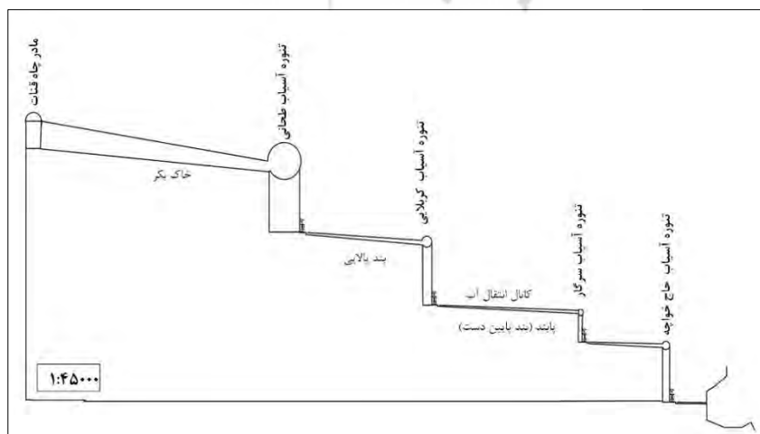
تصویر ۲۱. موقعیت قرارگیری چهار آسیاب روزمینی کشتخوان حنفش، بعد از مظهر قنات که با استفاده از ریخت طبیعی زمین که به صورت بند و پا بند می‌باشد در این کشتخوان ساخته شده اند منبع: نگارندگان، ۱۳۹۸
