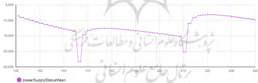
شکل ۱۵. کمبود مگاوات تولیدی نسبت به مگاوات مصرفی سناریوی ۲
