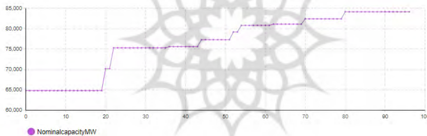
شکل ۳. ظرفیت اسمی اجرا مدل به مدت ۹۶ ماه
