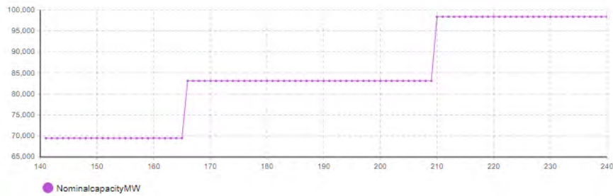
شکل ۱۴. ظرفیت اسمی سناریو ۲
