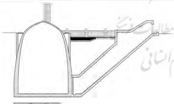
شکل ۱۲. برش از مخزن آب‌انبار دارکوب
