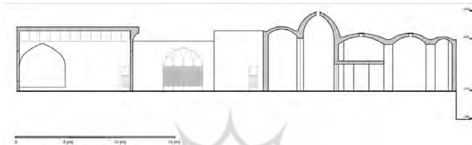
شکل ۸. برش عرضی از حسینیه ام‌البینین و رنگرزی گلپر
