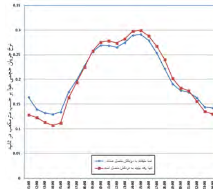
نمودار ۹- مقایسه جریان حجمی هوا در طبقه هفتم در دو حالت متفاوت.
