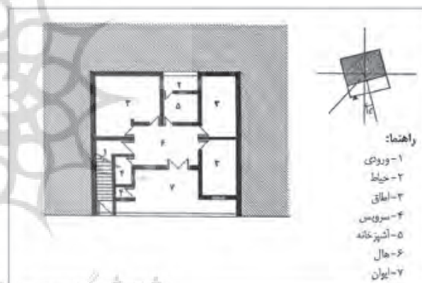
تصویر ۸- نمونه دوم خانه‌های تک‌خانوار غیر بومی (کوی طالقانی) مأخذ: (شرکت ماندان، تصحیح و تدقیق نقشه در سال ۱۳۶۶ توسط نگارنده)
