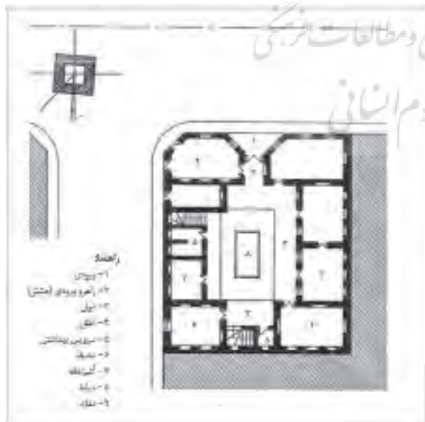
تصویر ۳- نمونه خانه تک خانواری (مستقل) بافت قدیم خرمشهر. مأخذ: (Ghaemian, تصحیح و تدقیق نقشه در سال ۱۳۶۶ توسط نگارنده)
