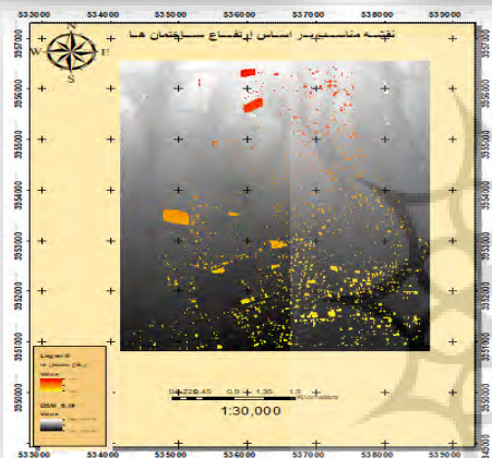
شکل ۳ نقشه های تولید شده معیارهای پنج گانه در مکان یابی پانل های خورشیدی - منبع نگارندگان
